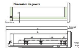
Dimensões da gaveta
